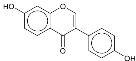
diadzein
